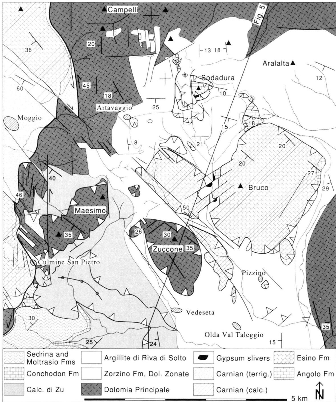
Fig. 4. Geological map of the Aralalta-Taleggio area.
