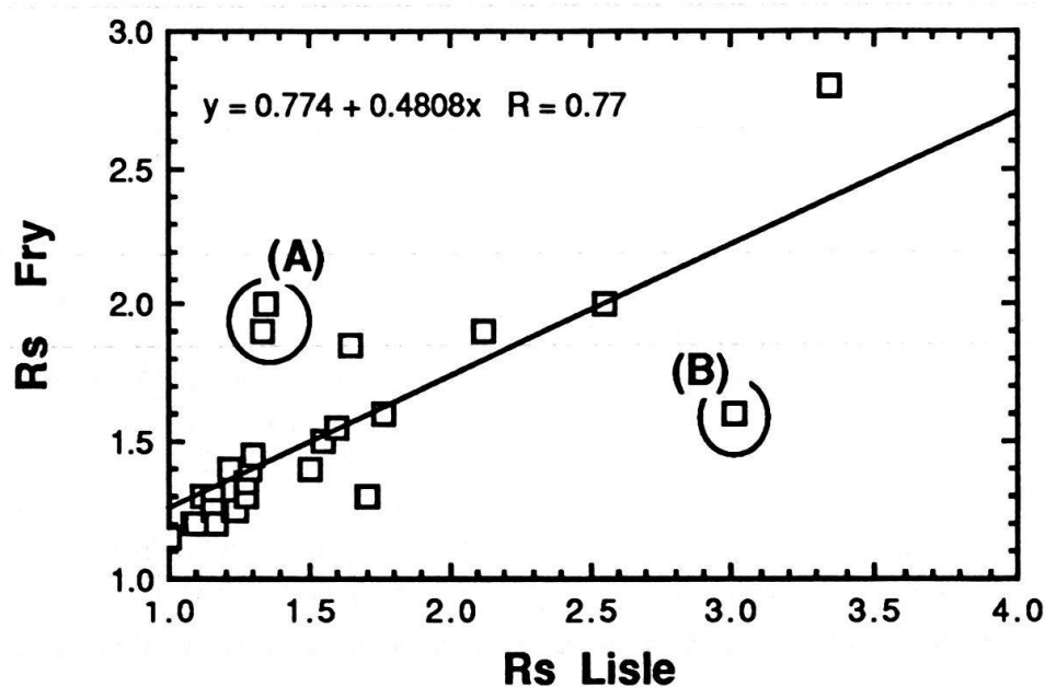
Fig. 4. Rapports de l'ellipse de déformation obtenus par la méthode R_f/\varnothing de LISLE et la méthode centre à centre de FRY. Sont inscrits dans le diagramme la corrélation linéaire et le coefficient de corrélation R. (A) et (B) réfèrent à des types de déformation décrits dans le texte.
