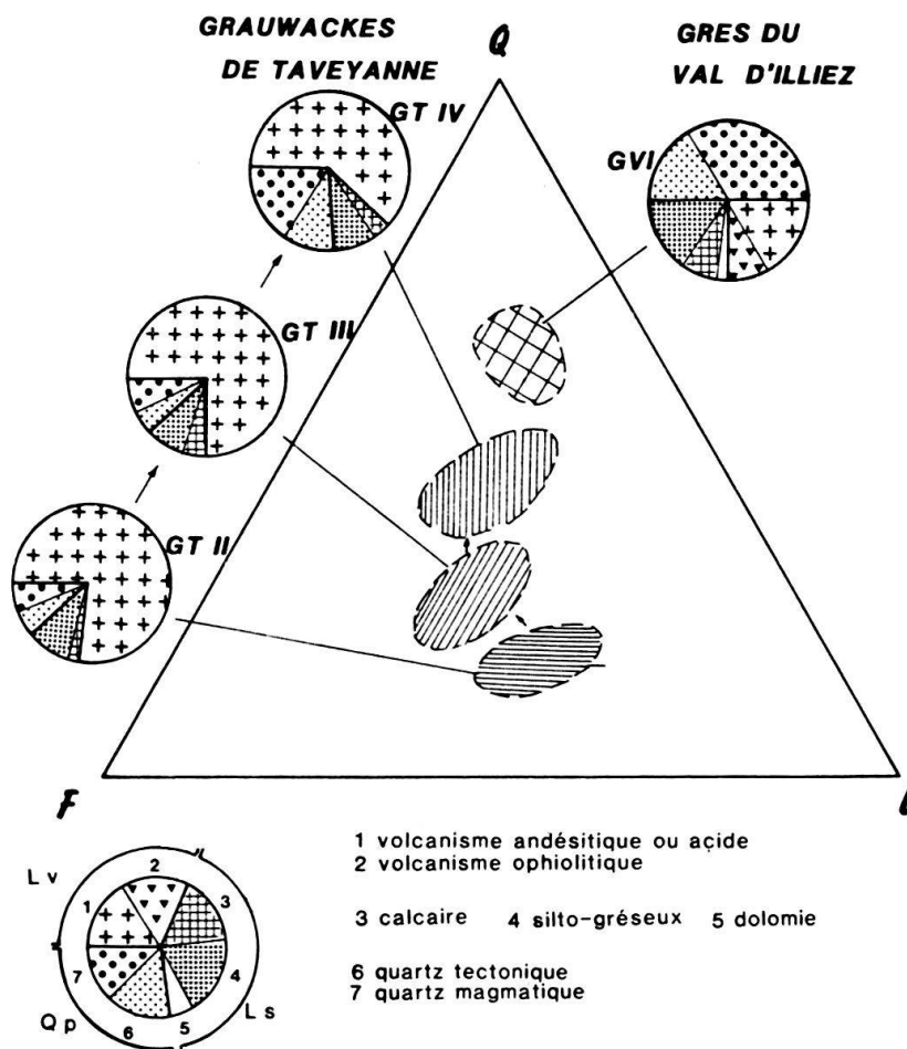
Fig. 4. Composition pétrographique des différents types de grauweekes (Grès de Taveyannaz), en comparaison avec celle des Grès du Val d'Illicz.
