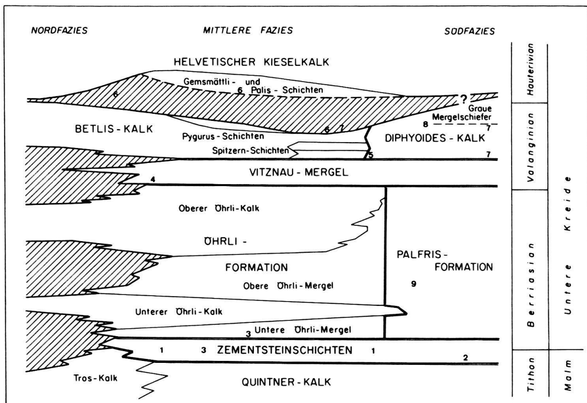
Fig. 1. Stellung der lithostratigraphischen Einheiten in der untersten Helvetischen Kreide. Die Darstellung ist schematisch; grössere Abweichungen westlich und östlich des Untersuchungsgebietes sind möglich. Formationsnamen sind gross, Namen von Formationsgliedern klein geschrieben. Hiatus und/oder Erosionsphasen sind schraffiert dargestellt. In der Vertikalen ist die Zeit maßstäblich aufgetragen, deshalb macht die Skizze keine Aussagen über Schichtmächtigkeiten bzw. Sedimentationsraten. Datierungspunkte: 1: DIEGEL (1973), 2: ARN. HEIM (1907), 3: SCHINDLER (1959), 4: PANTIĆ & BURGER (in Vorb.), 5: ARN. HEIM (1916), 6: HALDIMANN (1977), 7: ISCHI (1978), 8: STRASSER (1979), 9: TOBLER (1899b).
