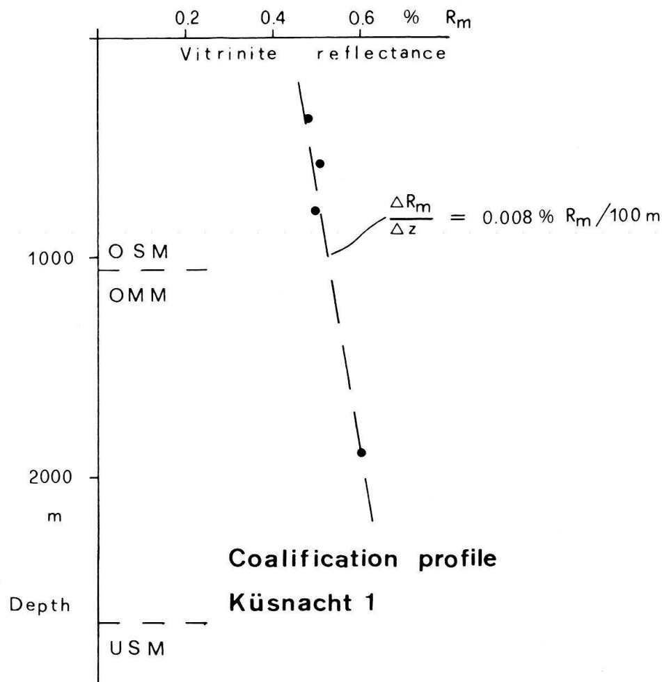
Fig. 6. Das Inkohlungsprofil der Bohrung Küsnacht 1 ZH ist charakterisiert durch niedrige Inkohlungswerte ( <0,6\% R_m ) sowie durch ebenfalls niedrigen Inkohlungsgradienten. USM = Untere Süsswassermolasse, OMM = Obere Meeresmolasse, OSM = Obere Süsswassermolasse.
