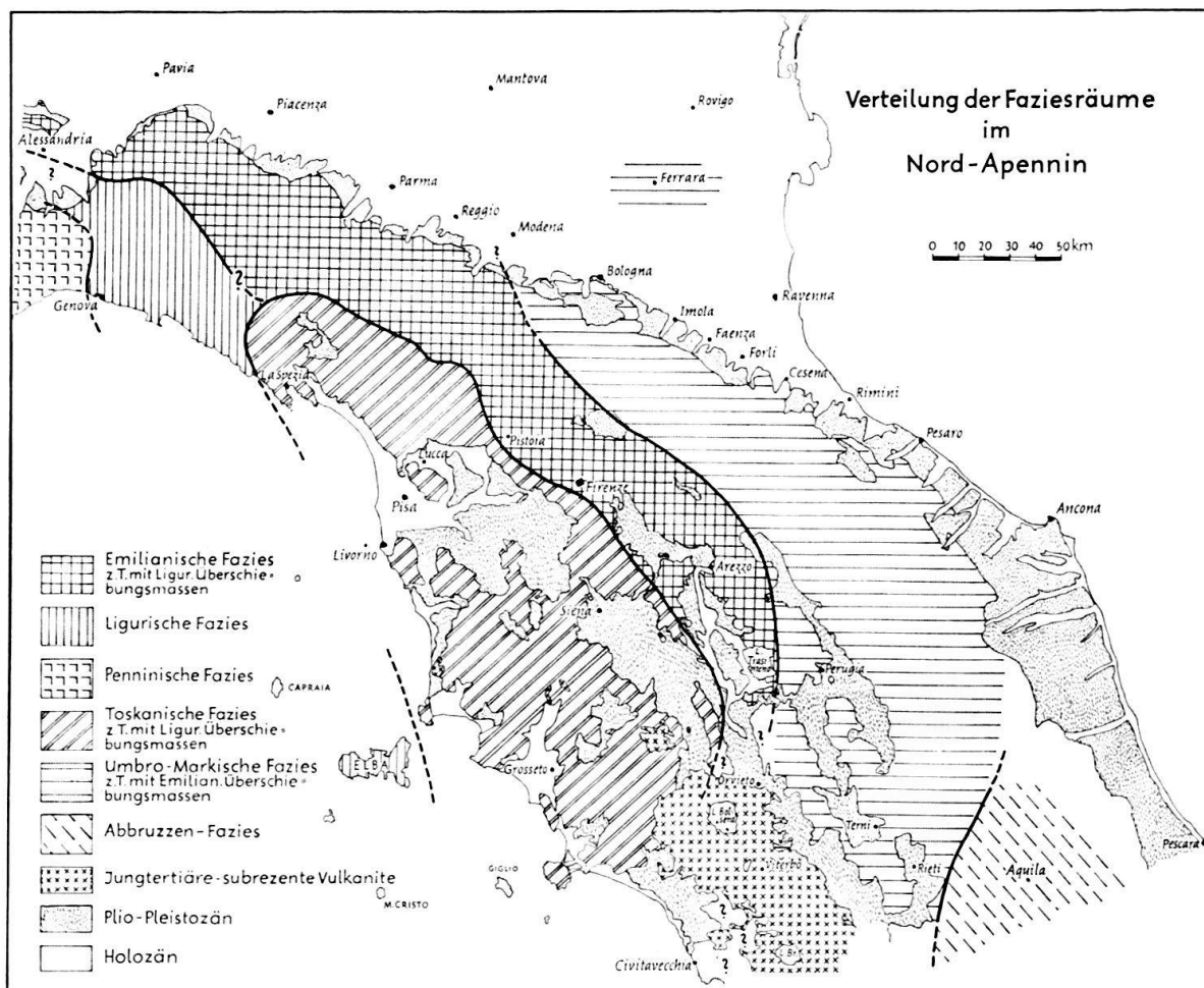
Fig. 4. Verteilung der Faziesräume des Nordapennins unter der Voraussetzung, dass ein externer Emilianischer Eugeosynklinaltrug existiert.
