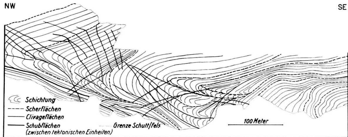
Fig. 3. Detail aus der Nordostflanke des Limmernbodens. (Ochsenplanggen der Karte Oberholzer, Lit. 4), Strukturen und Clivage im Unteren Quintnerkalk. Geologischer Aufriss 1:5000.
