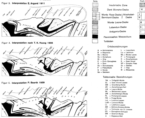
Figur 3-5 Tektonisches Profil durch die Weissries-Gruppe 1:400.000
