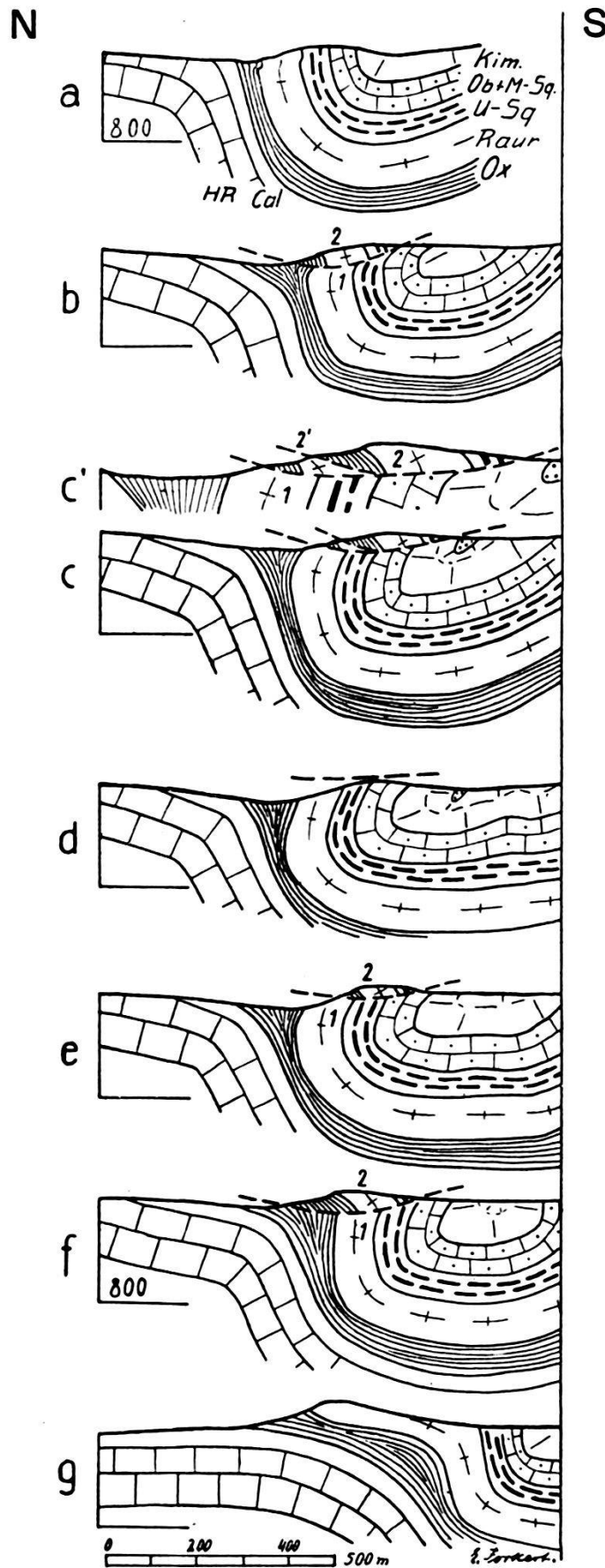
Flankenüberschiebung im Südschenkel der Rameaux-Kette östlich Les Rouges Terres. (Profil c' ist die zweifache Vergrößerung von Profil c.)
