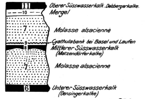
Gliederung der stampischen Glimmermassen.
