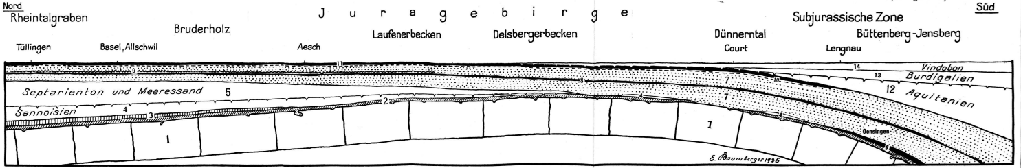
1. Mesozoische Unterlage. 2. Balmzerformation (eocaen). 3. Buchsweiler-Planorbentkalk (eocaen). 4. Sannoisien. 5-11. Stampien. 12. Aquitaniens. 13. Burdigalien. 14. Vindobonien [Helvetien und Tortonien (Silvaneschichten)]
