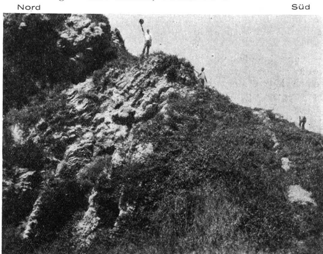
Fig. 3. Mergel mit Orthophragminen und Lepidocyclinen (Priabonien = Jacksonstufe) B 4 und tiefste Bänke von C (vgl. Fig. 2). Einfallen ca. 50° nach N.
