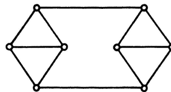
E=8 ; F_3=4 , F_6=2
