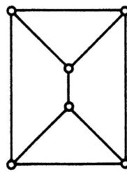
Figur 5. E=6 ; F_3=2 , F_4=3 .
