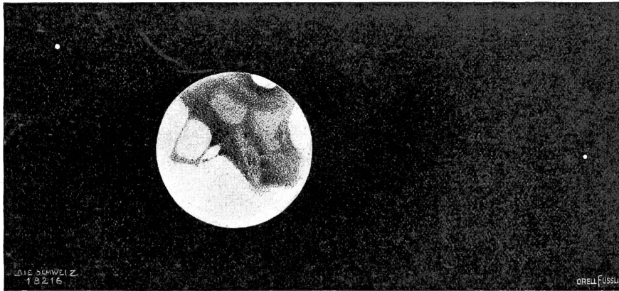
Bild des Mars mit seinen beiden Monden (wiedergegeben nach G. M. Antoniadi im Bulletin der Société Astronomique de France, mit Ermächtigung dieser Gesellschaft und des Herrn Antoniadi). Das Bild zeigt, wie wenig deutlich man den Mars im günstigsten Falle sehen kann.
