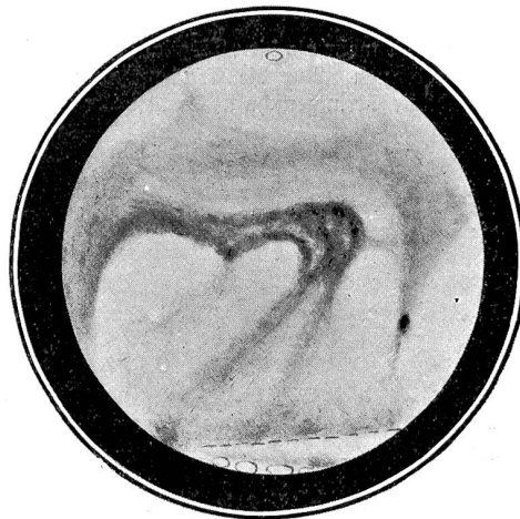
Marsbild am 4. Nov. 1911 von J. Comas Solá in Barcelona, Präsident der Sociedad Astronómica de España, mit dessen Ermächtigung aus der Vereinszeitschrift wieder gegeben. Der mittlere Teil dieses Bildes, die Gebirgslandschaft des Sinus Sabaeus darstellend, bedeutet einen Triumph des menschlichen Auges. Der Küste des hellen Meeres entlang bezeichnet zunächst ein dunkler Streifen die schneebedeckte Seite eines Gebirgszuges; dann folgt eine Reihe heller Flecken, die Schneefelder auf der andern Seite des Gebirgszuges; hierauf eine unregelmäßige Verteilung von hell und dunkel und nach rechts oben wieder ein dunkler Abhang; die zugehörige schneebedeckte Seite verschwindet mit der Schneedecke eines breiten Tales. Es ist zu beachten, daß der Mars nur halb so deutlich zu sehen war wie 1909 und daß Herr Comas Solá diese Zeichnungen veröffentlichte, bevor er meine Erklärung angenommen oder auch nur gefasst hat.
