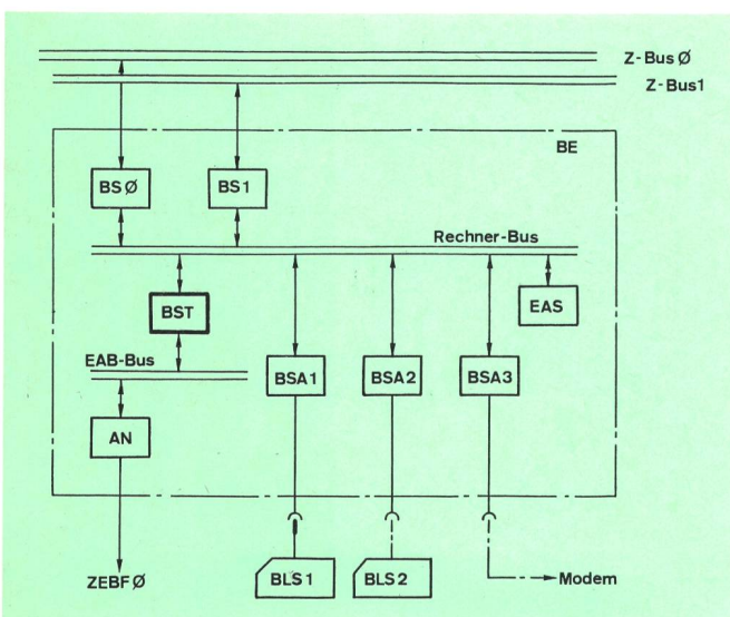
Fig. 6 Bedieneinheit A 52 S/HS 52 B AN Anschalter BST Bedieneinheitssteuerung EAB-Bus Ein-/Ausgabe-Bausteinbus ZEBF Zentraleinheit-Bedienungs-feld (Weitere Abkürzungen siehe Text)
