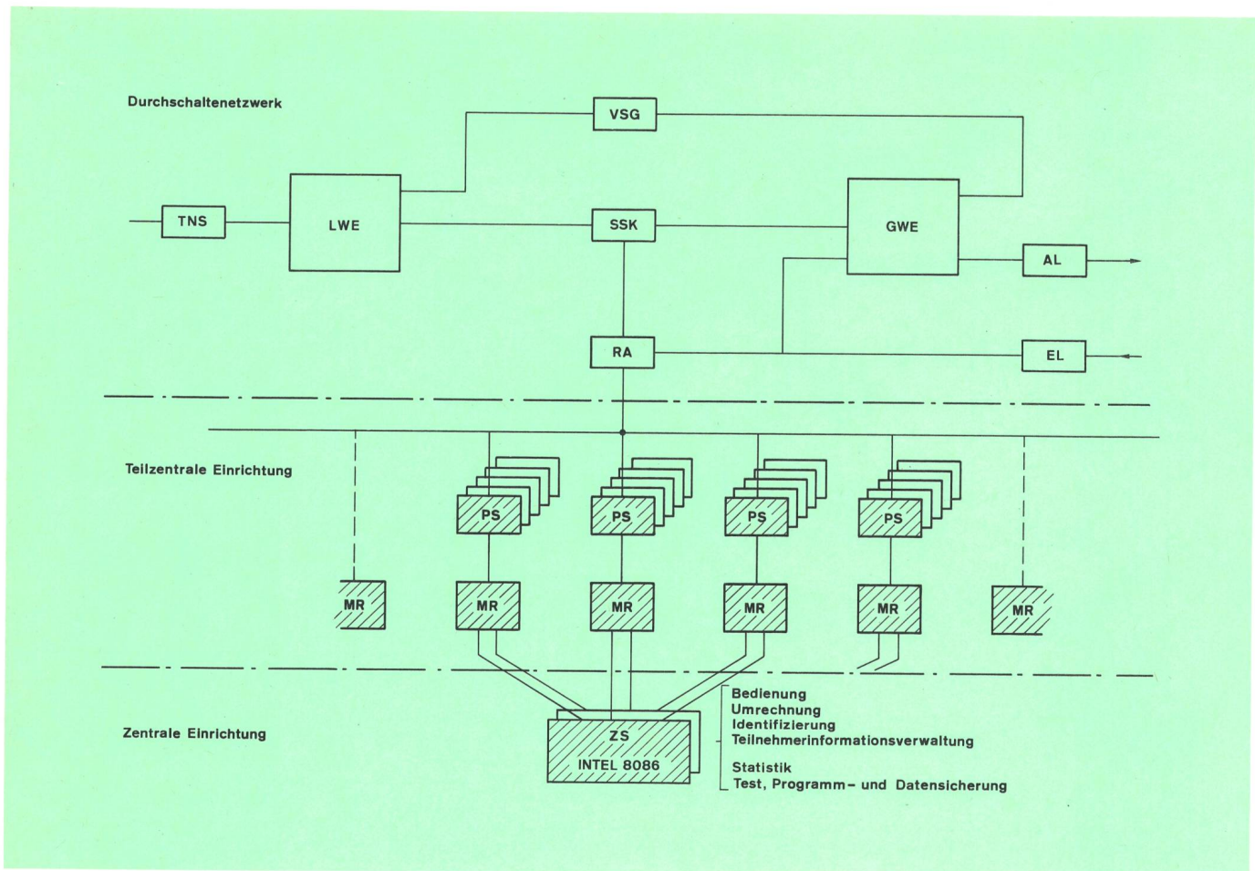
Fig. 10 Blockscheema einer Pentaconta-Ortszentrale mit SPC-Register (PC 85)
