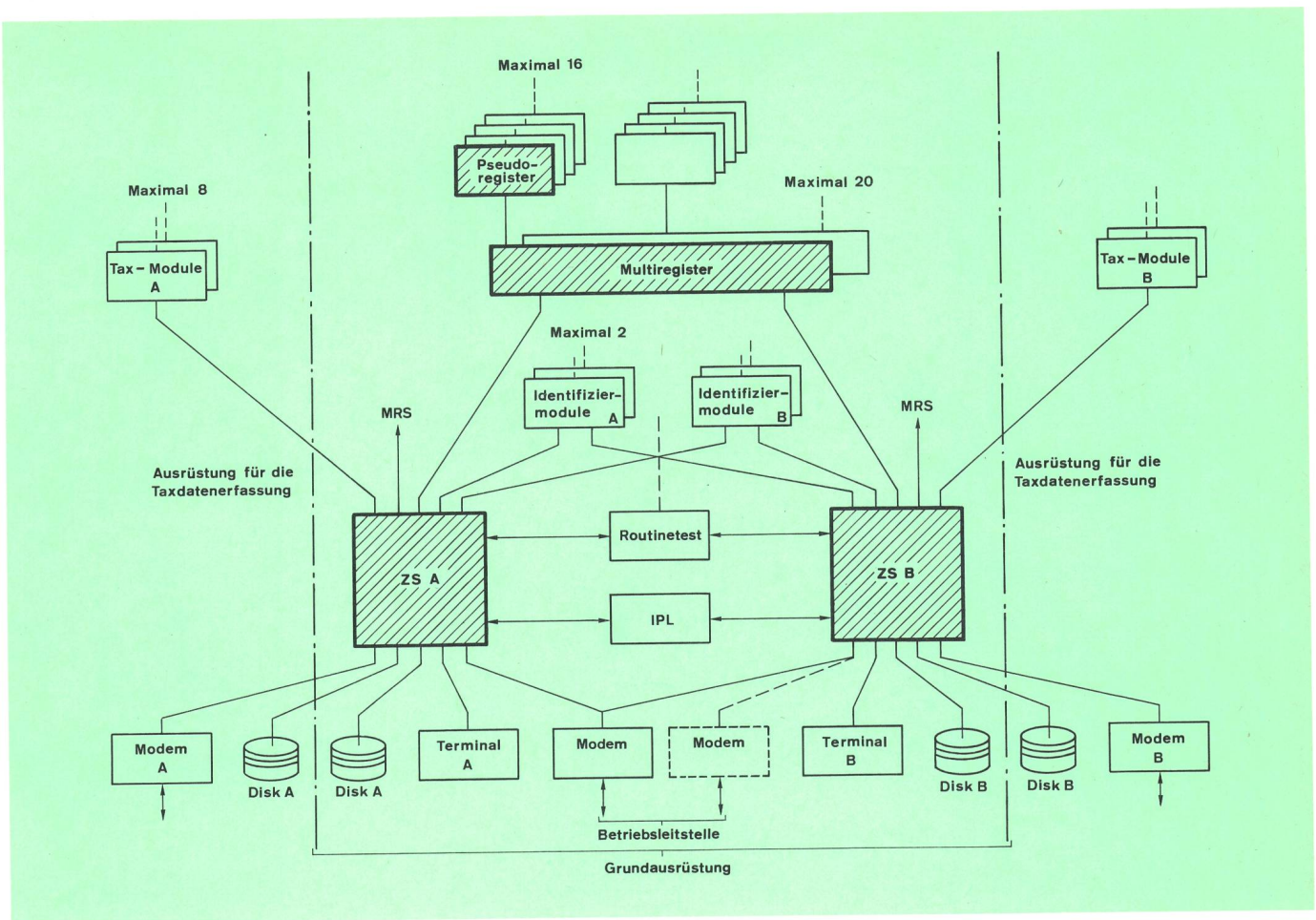
Fig. 11 Prinzipieller Aufbau der SPC-Register IPL Interprozessoren-Link MRS Meldungs-Registrierungs- und Statistik-Einheit
