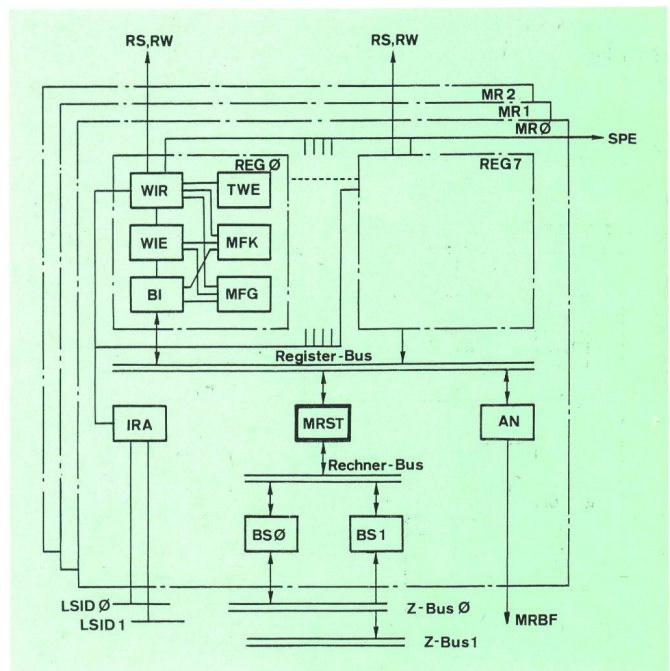
Fig. 5 Multiregister A 52 S AN Anschalter IRA Identifiziererringanschlaltung LSID Leitungssystem des Identifizierers MRBF Multiregister-Bedienungsfeld REG Register SPE Rechnergesteuerte Prüfeinrichtung für Register Z-Bus Zentralbus (Weitere Abkürzungen siehe Text)
