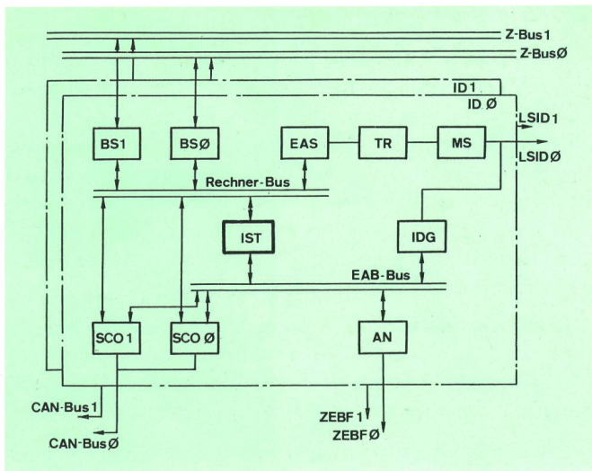
Fig. 4 Identifizierer A 52 S/HS 52 B CAN-Bus Codieranschaltebus EAB-Bus Ein-/Ausgabe-Bausteinbus MS Minusschalter TR Trenner Z-Bus Zentralbus (Weitere Abkürzungen siehe Text)
