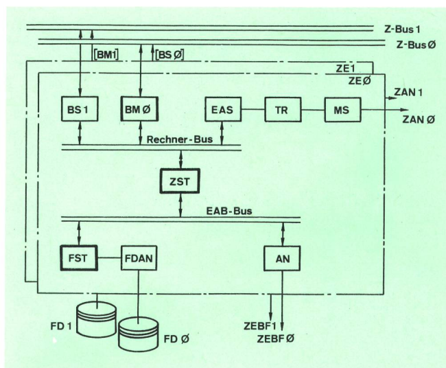
Fig. 3 Zentraleinheit A 52 S/HS 52 B MS Minusschalter TR Trenner ZAN Potentialanschl. (in der Zentraleinheit) ZST Zentraleinheitssteuerung (Weitere Abkürzungen siehe Text)
