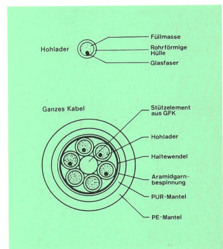
Fig. 1 Aufbau des Glasfaserkabels der optischen Übertragungsstrecke Altdorf—Erstfeld
