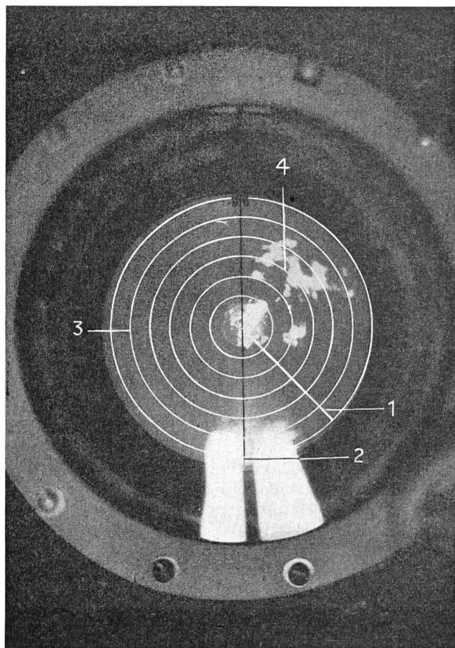
Fig. 6. Leuchtschirm der PPI-Röhre (Plan and Position-Indicator)
