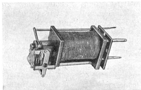
△-Relais „Bell“
