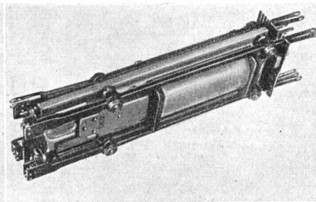
Flachtyprelais „Hasler“
