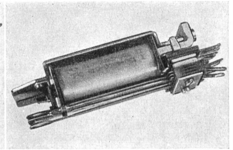
Flachtyprelais „Siemens“
