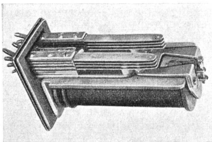
Eriksonrelais „Hasler“
