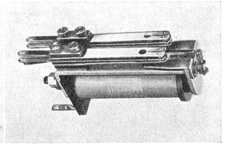
Normalrelais „Gfeller“
