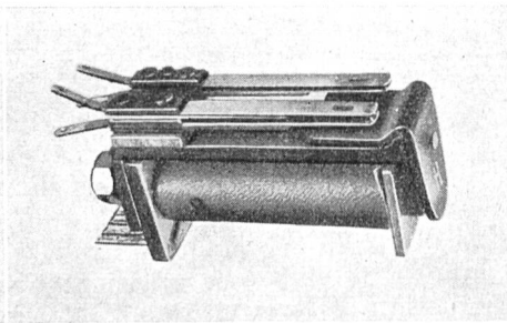
Schneidankerrelais „Siemens“
