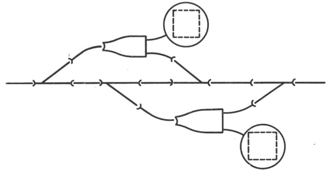
Fig. 2 Anordnung für 2 Pupinspulen Disposition pour 2 bobines Pupin
