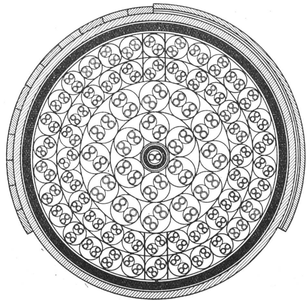
Fig. 3. Querschnitt des Kabels mit 72 Vierern.
