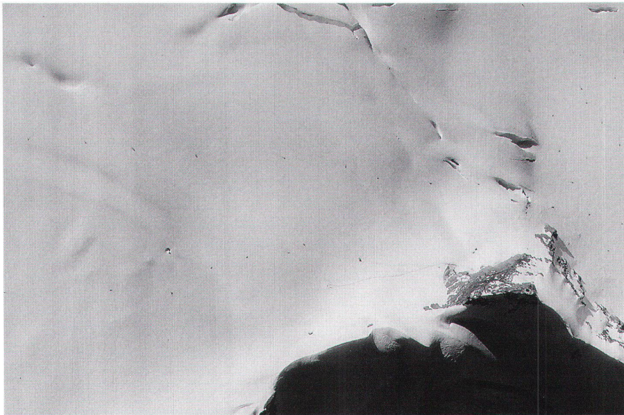
Abb. 10: Ein Gletscher mit «Laubflecken»: Damit der Aletschgletscher überhaupt photogrammetrisch ausgewertet werden konnte, musste er zuerst künstlich mit über 10 000 Punkten aus Sägemehl und Russ versehen werden. Ausschnitt einer Partie auf dem oberen Jungfraufirn südlich der Sphinx (Photothek L+T, Aufnahme 4077 aus der Fluglinie 3a / ALETSCHE vom 20. 8. 1957). Der Mönch selbst wies genügend Kontrast auf und musste nicht zusätzlich «getupft» werden.
