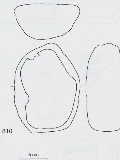
Onnens VD- Le Motti . Mobilier de la zone marécageuse. Bronze (éch. 1/1). 805: anneau. Terre cuite (éch. 1/4). 806: croissant. Bois de cerf (éch. 1/2). 807-808: andouillers. Pierre (éch. 1/4). 809-810: matériel de mouture. 811: galet encoché.
