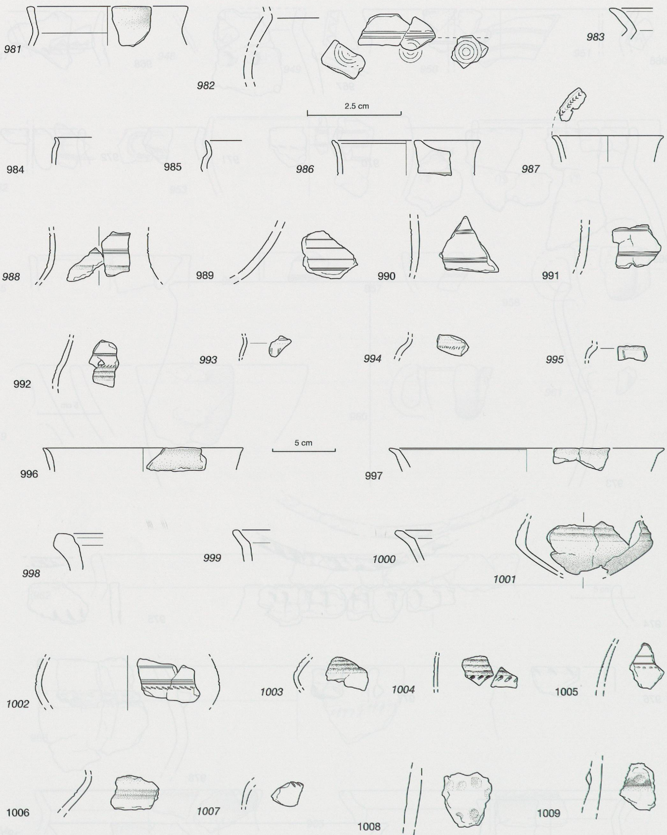
Onnens VD-La Golette (éch. 1/3 et 1/1). 981-985: pots en pâte fine ou moyenne. 986-995: gobelets à épaulement. 996-1000: bords. 1001-1009: panses décorées.
