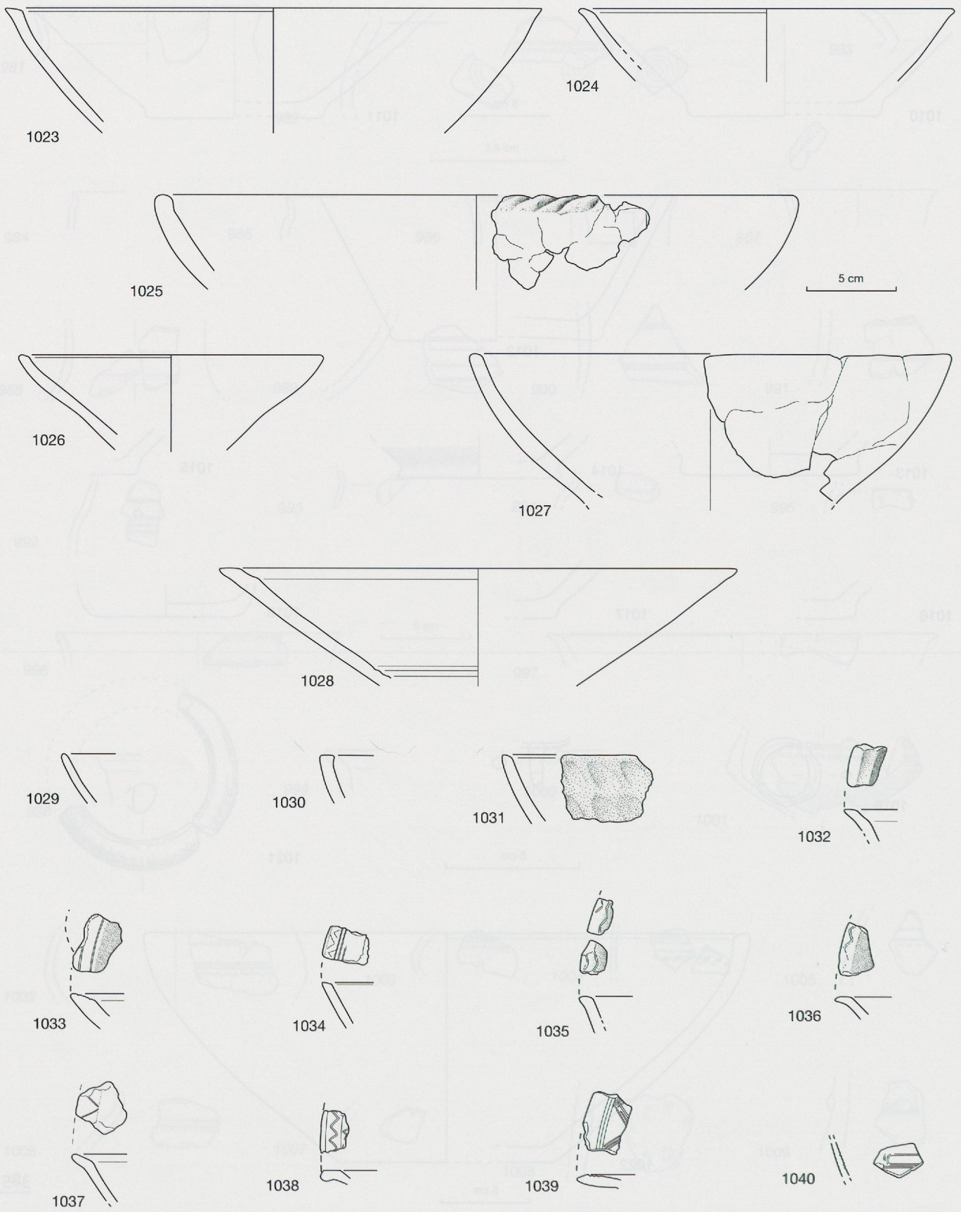
Onnens VD-Beau Site (éch. 1/3). 1023-1040 : écuelles.
