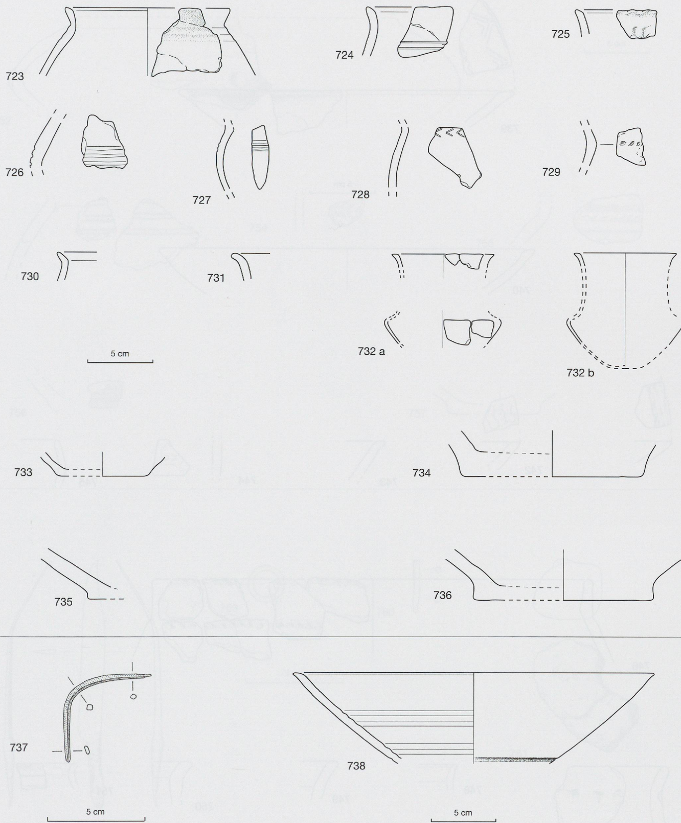
Onnens VD- Le Motti . (éch. 1/3). 723-731: pots en pâtes moyenne et fine. 732 (a): gobelet à épaulement. 732 (b): reconstitution. 733-736: fonds. Mobilier du versant de la colline. Bronze (éch. 1/1). 737: ciselet. Céramique (éch. 1/3). 738: écuelle.
