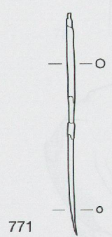
Onnens VD-Le Motti (éch. 1/3). 767: pot en pâte grossière. Mobilier de la solifluxion. Bronze. 768: épingle (éch. 1/1). 769-771: épingles (éch. 1/2). 772: poinçon (éch. 1/1).
