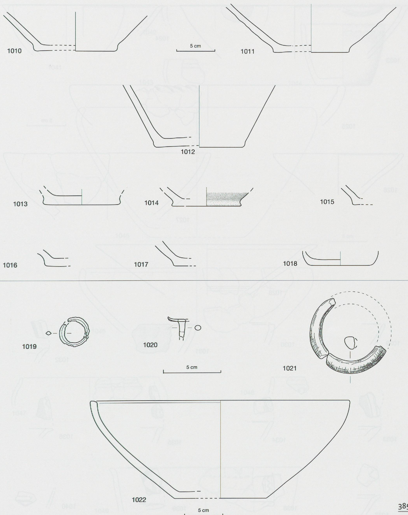
Onnens VD-La Golette (éch. 1/3). 1010-1018: fonds. Onnens VD-Beau Site. Bronze (éch. 1/2). 1019: anneau. 1020: épingle. Schiste bitumineux (éch. 1/2). 1021: bracelet. Céramique (éch. 1/3). 1022: écuelle.
