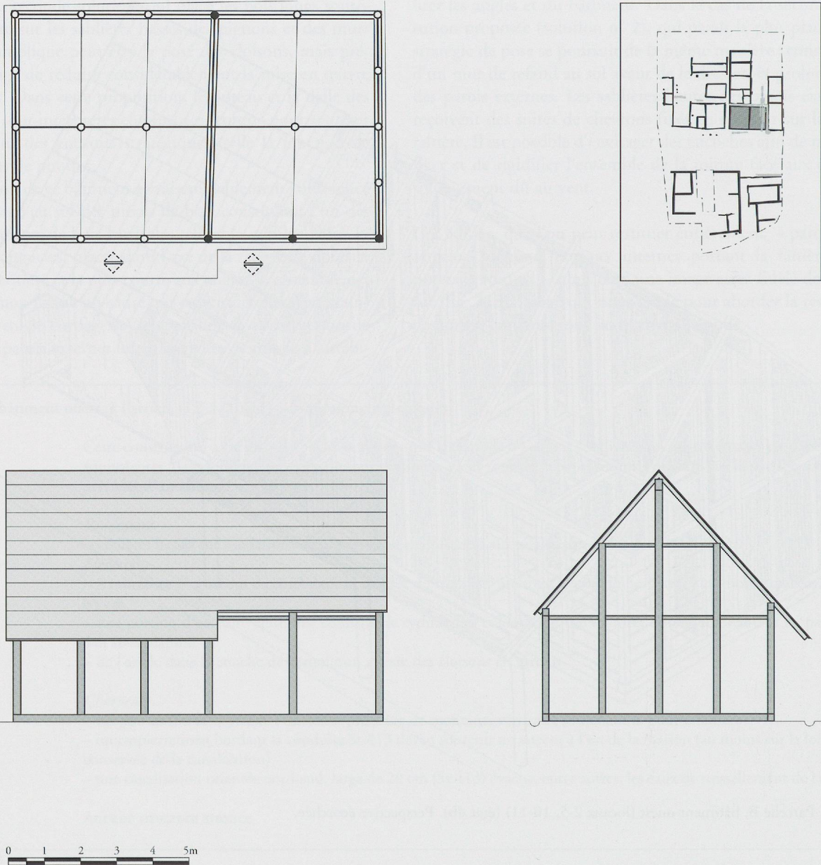
Fig. 219. Parcelle B, bâtiment avant (locaux 1 et 12) (état 4b). Type : à deux pièces. Plan et élévations schématiques. Pour les conventions graphiques, se reporter à la fig. 217.
