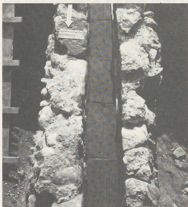
Fig.28. Zone B: canalisation 312, tronçon nord (état 3B).
