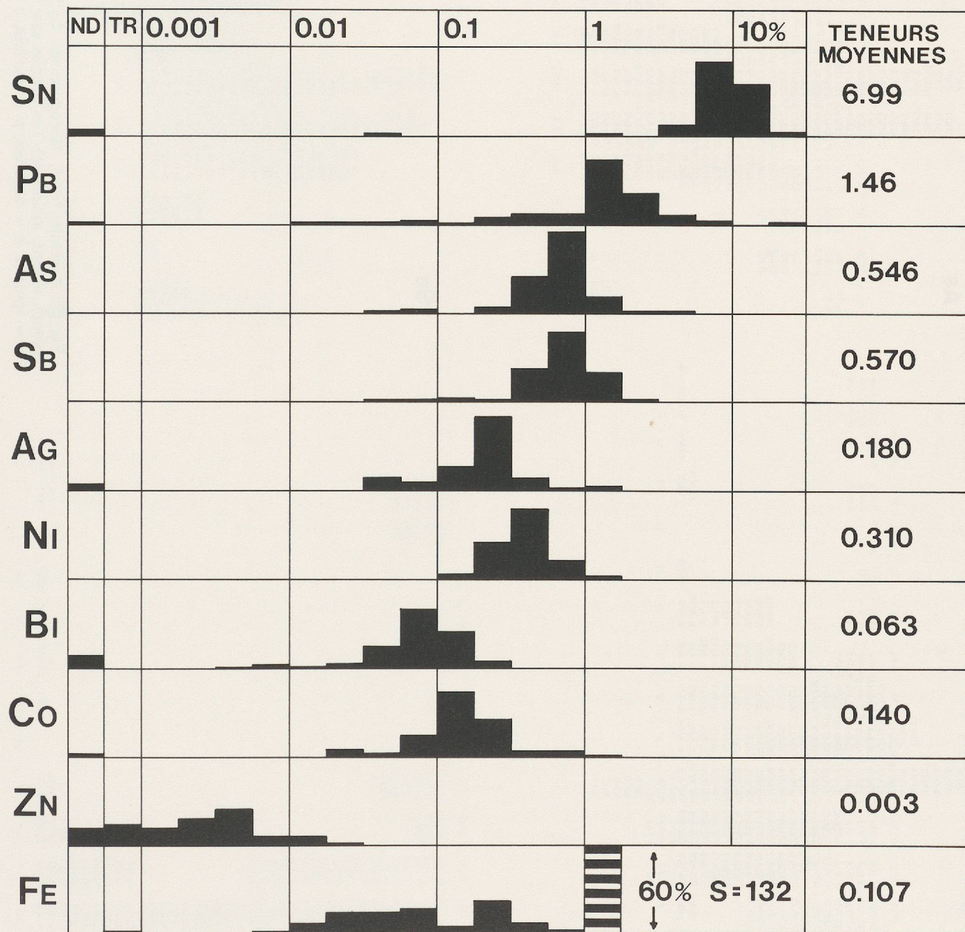
Fig. 4 Auvergnier/Nord. Diagramme des analyses de bronze, d'après le modèle proposé par Waterbolk et Butler (1965). Les intervalles sont les suivants (échelle logarithmique): ND = non détecté TR = traces
