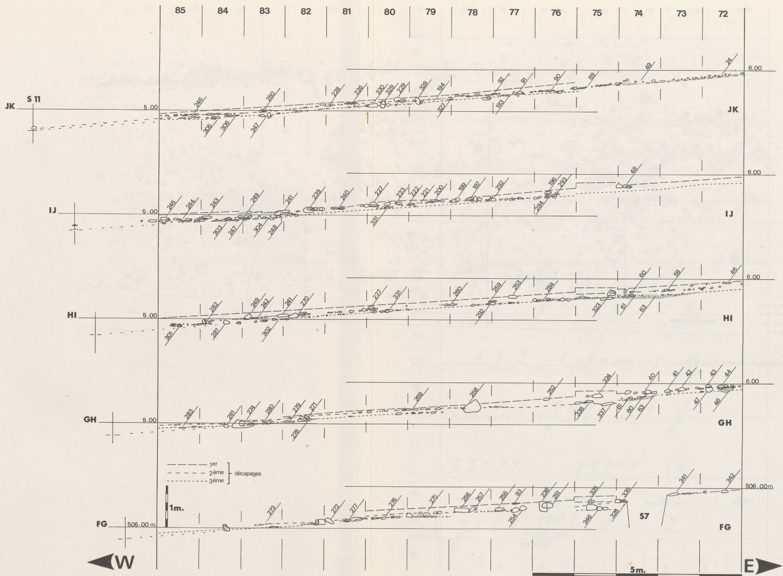
Figure 128 Coupes théoriques est-ouest dans le secteur FL/71-85.
