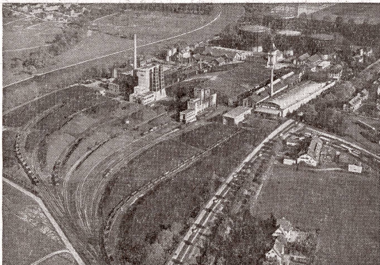
Oben: Flugbild des Gaswerks Zürich, des größten Kohlenveredelungsbetriebes unseres Landes. Im Vordergrund die Kohlenlager, im mittleren Bildabschnitt die Aufbereitungs- und Produktionsanlagen und im Hintergrund die Gasbehälter.
