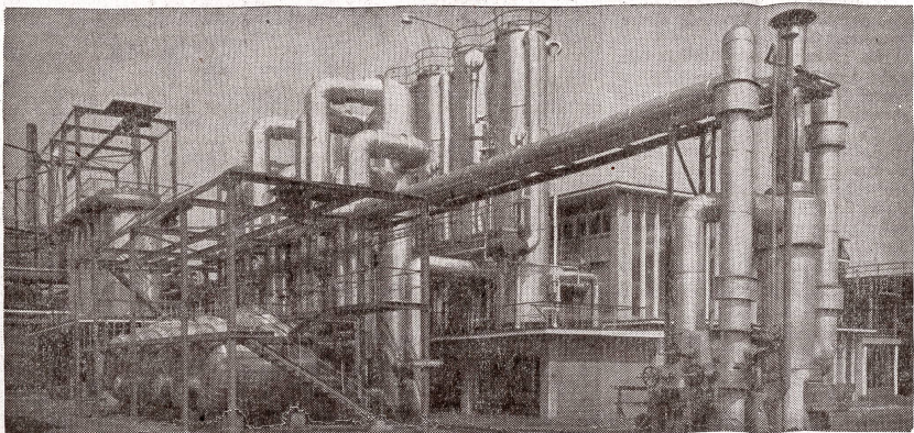
Unten: Die Gasentgiftungsanlage des Gaswerkes Basel mit den waagrecht liegenden Reaktoren (linker Bildabschnitt), den Sättigern und Kühlern (senkrechte Türme) und dem Apparatehaus (rechts im Hintergrund).
