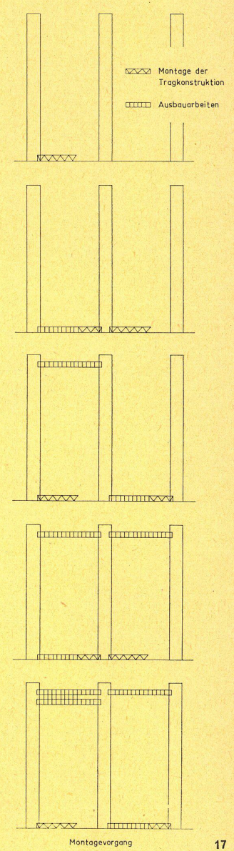
Montagevorgang
