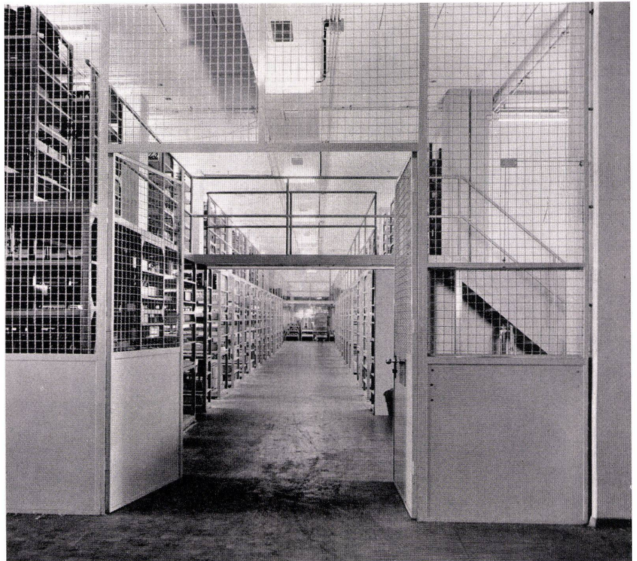
3 Lager im Erdgeschoß des Flachbaus. Kopflose Stahlbetonpilzdecke. Magasins au rez-de-chaussée du bâtiment plat. Dalle-champignon. Stores on ground floor of flat building. Headless reinforced concrete mushroom ceiling.
