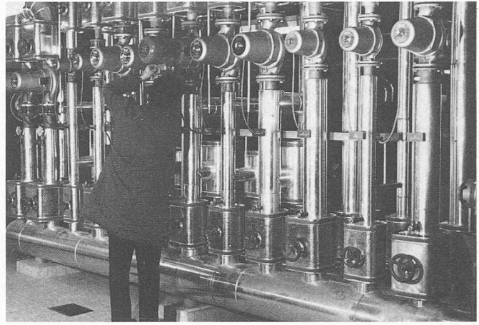
Fig. 24. — Distributeur — collecteur avec groupes prérégés.
