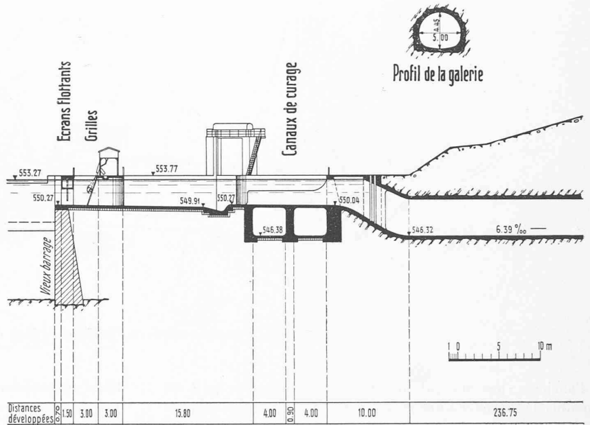
Fig. 3. — Usine hydro-électrique de l'Oelberg. — Coupe en long de la prise d'eau.
