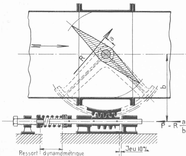
Fig. 5. — Schéma d'un dispositif pour mesurer les poussées hydrauliques sur un papillon.
