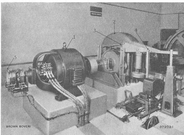
Fig. 5. — Commande du treuil de la station de Weissfluhjoch. 1 = Moteur principal. — 2 = Engrenage réducteur principal. — 3 = Frein de service à commande par électro-aimant et à main. — 4 = Frein automatique de secours (levier à droite). — 5 = Interrupteur à force centrifuge.
