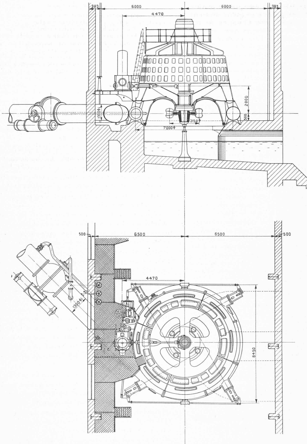
Fig. 1. — Turbine Pelton à axe vertical de Maipo. Echelle 1 : 150.
