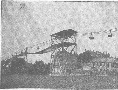
Chemin aeri « Bleichert » pour une usine electrique.
