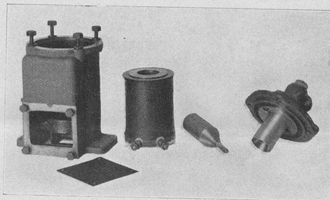
Fig. 16. — Valve du frein d'alarme.
