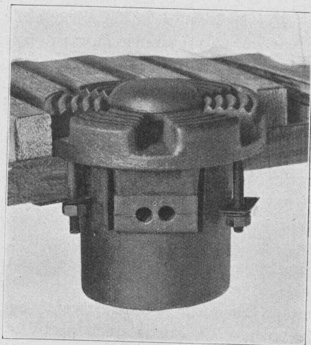
Fig. 15a. — Pédale de sécurité. — Ensemble.
