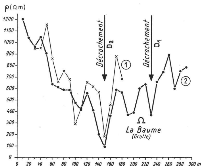
Fig. 6. Profils géoélectriques exécutés à l'aide d'électrodes de courant fixe (Fixed Current Electrode Array: FCE). 1 = AB 200 m; 2 = AB 500 m. MN = 10 m. Les profondeurs d'investigation sont respectivement de 20 et 50 m au moins.
