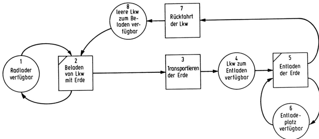
Figur 2. Die Erdbewegungsoperationen als Skizze und Modell
