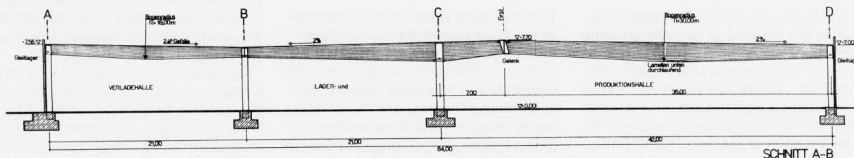
Bild 2: Schnitt
