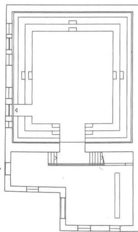
Grundriss Erdgeschoss
