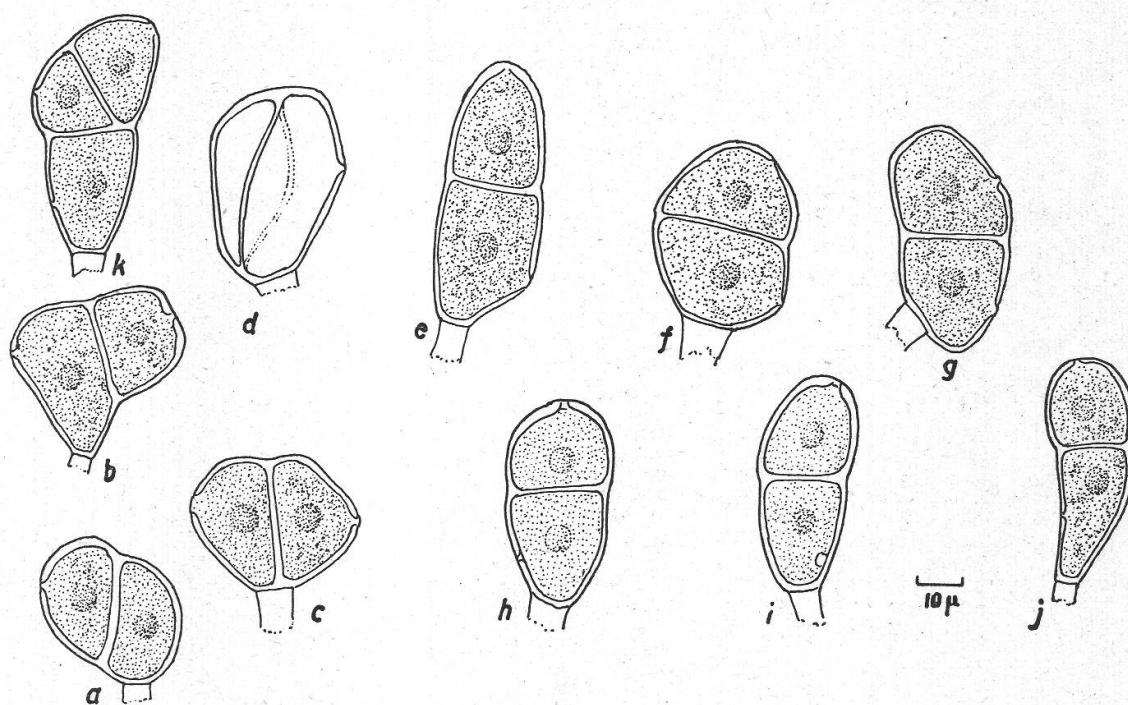
Figure 6 Diverses formes de téliospires. Voir texte
