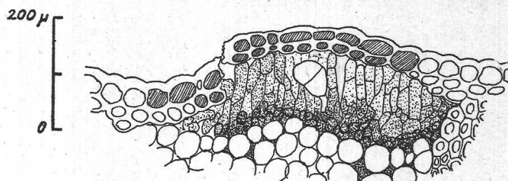
Figure 2 Une téliosore jeune hyaline apparaît au sein du stroma. Epiderme et hypoderme nécrosés
