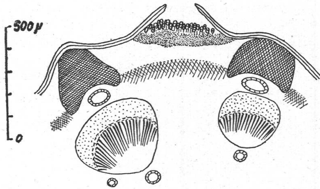
Figure 4 Localisation d'un téliosore pétio- laire entre deux piliers de scléren- chyme. Le stroma est en grisé, dans le parenchyme chlorophyl- lien limité intérieurement par la gaine interfasciculaire de tissu sclérifié
