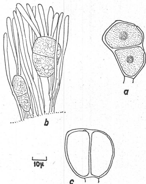
Figure 10 Puccinia bullata (Pers.) Wint. sur Conium maculatum L. a télis- spore, b télisporés naissantes dans un sore mixte à paraphyses; c télisporé à cloison verticale. Echantillon B r i o s i et C a v a r a n° 210.
