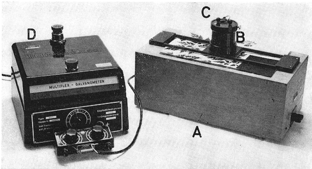
Abb. 2. Detailphotometer (Hersteller Dr. B. Lange, Berlin). A Lichtkasten, innen der Lampenkrantz, B Messtube, C Photoelement, D Messgerät.
