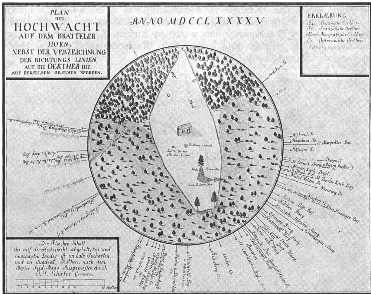
Bild 5. Hochwacht auf dem Prattler Horn, datiert 1795. Nach dem Plan von J. J. Schaefer. Zu beachten ist die abgeholtzte und eingehagte Parzelle mit «Holtz Piramiden zum Allarm Feur», Mörser, Richtungsscheibe und Wachthauslein.
