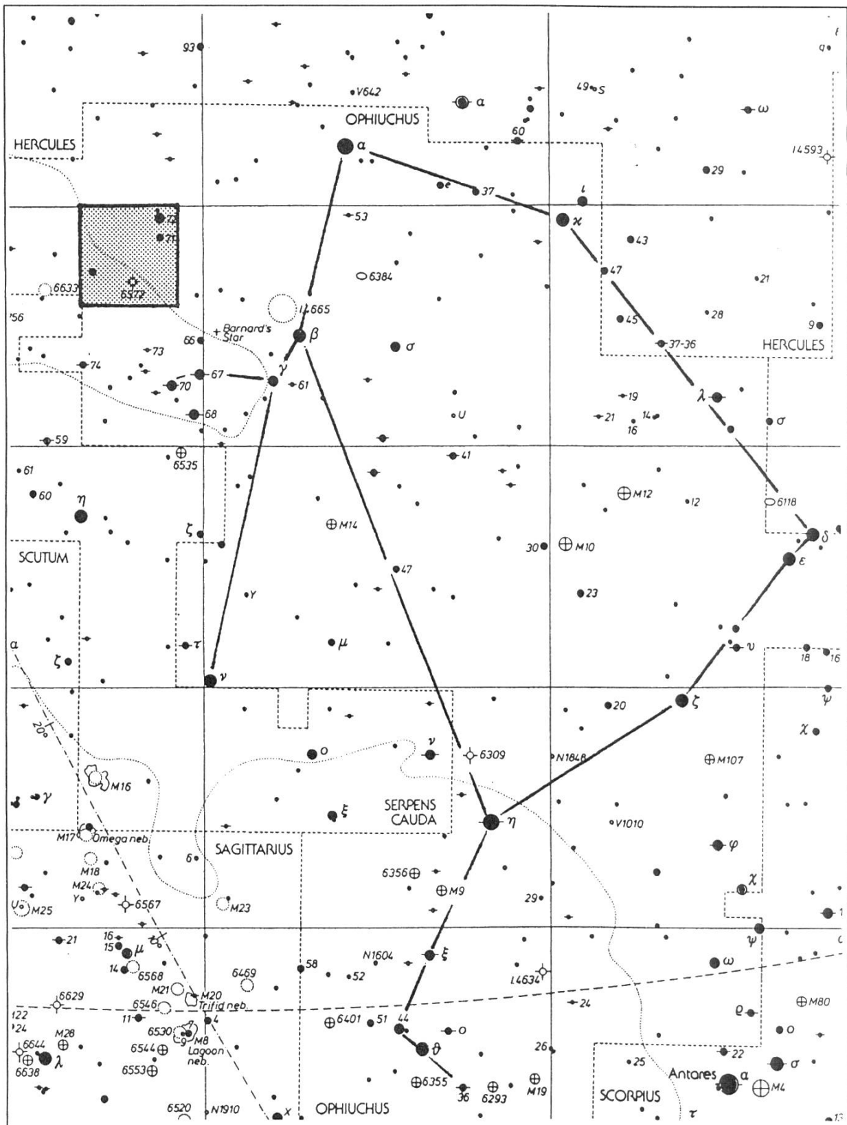
Abb. 3: Umgebungskarte für NGC 6572. Das Objekt liegt im schraffierten 4 \times 4^\circ -Feld (siehe auch Abb. 4). Aus dem Cambridge Star Atlas 2000.0. Mit freundlicher Genehmigung des Verlags.
