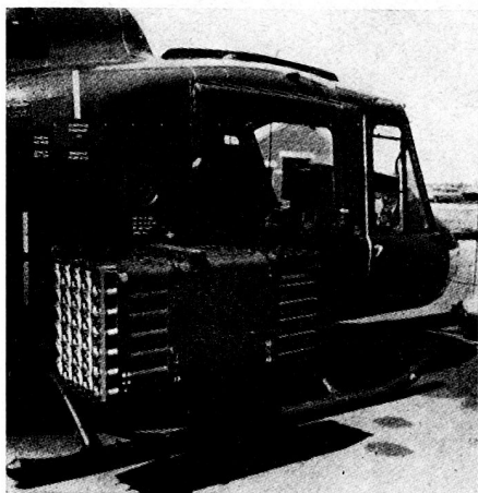
Bild 3. Lufraketenwerfer XM3 mit Spezialausrüstung für das Abfeuern von 288 AN-M8-Nebelskörpern vom Helikopter aus. In Höhen zwischen 60 und 90 m kann bei einer Geschwindigkeit von 75 bis 140 km/h ein 1000 m langer Nebelgürtel gelegt werden.
