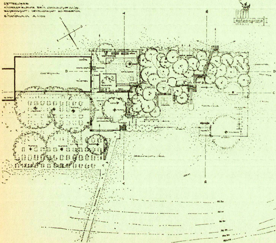
Grundriss des Projektes im 1. Rang von Walter Frischknecht, Gartenarchitekt BSG, Zürich. Ausführliche Beurteilung des Projekts siehe unter «Das Ergebnis der Beurteilung» im Text.
