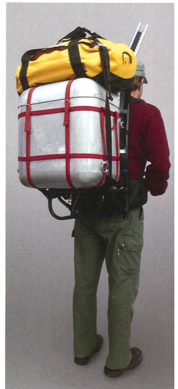
Fig. 2 : Prototype de caisson isotherme et équipement fixés sur un Tatonka® Lastenkraxe.
