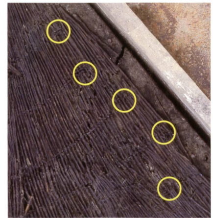
Abb. 44 Cham, Bibersee. Reuse Pos. 134, Innenseite. Die hintereinanderliegenden Rundenschlüsse (gelbe Kreise) auf einer Seite der Reuse sind gut sichtbar.
