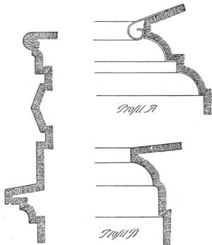
Schnitt A. B. durch die Erdschloßfensterbrüstung. — Maßstab 1:10
