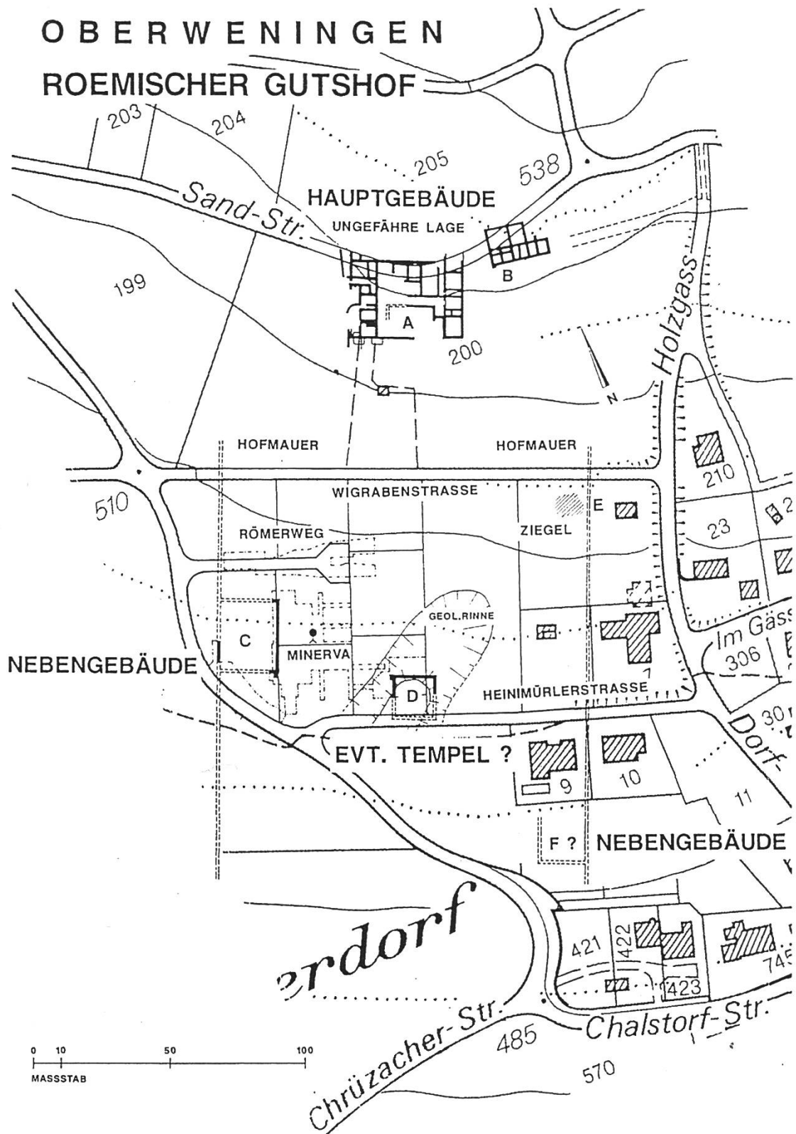
Abb. 1: Oberweningen ZH, Heinimürler. Provisorischer Gesamtplan des römischen Gutshofes. Plan Kantonsarchäologie Zürich
