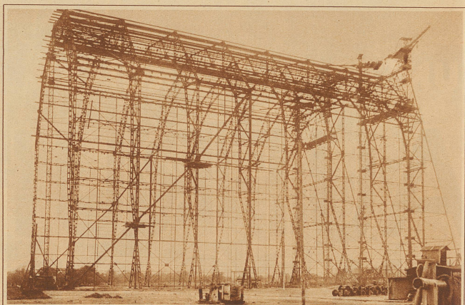
Die größte Luftschiffhalle der Welt mit 900 000 Kubikmeter umbautem Raum ist gegenwärtig in Friedrichshafen im Bau begriffen. Sie soll schon im März nächsten Jahres fertig sein und zur Aufnahme des neuen riesigen Zeppelinluftschiffes dienen
